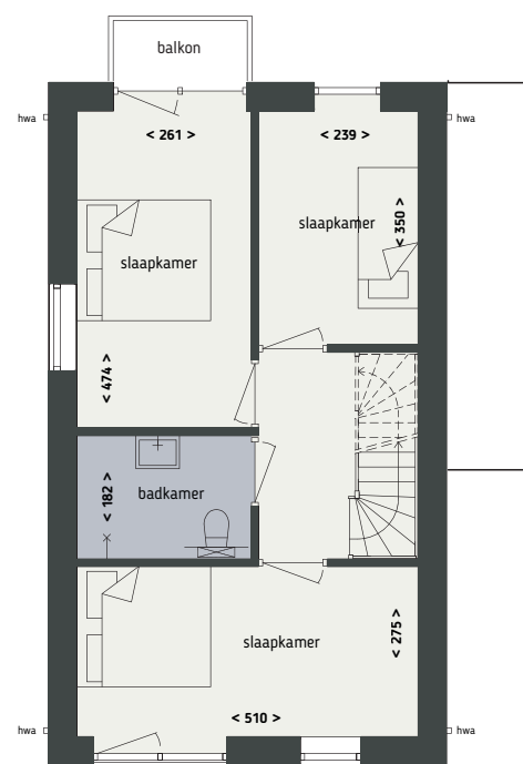
EERSTE VERDIEPING
