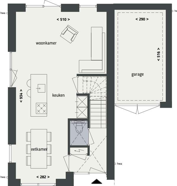
BEGANE GROND
