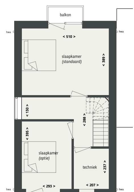
EERSTE VERDIEPING
