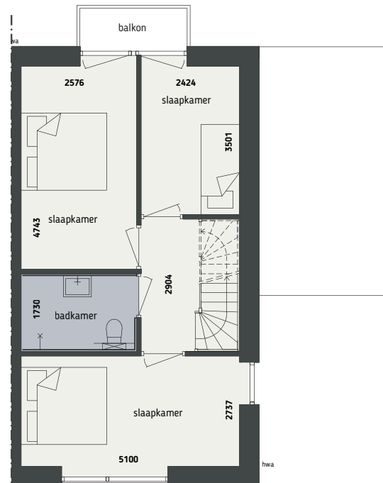
EERSTE VERDIEPING
