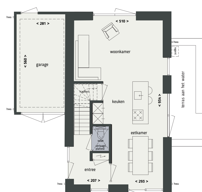
BEGANE GROND
