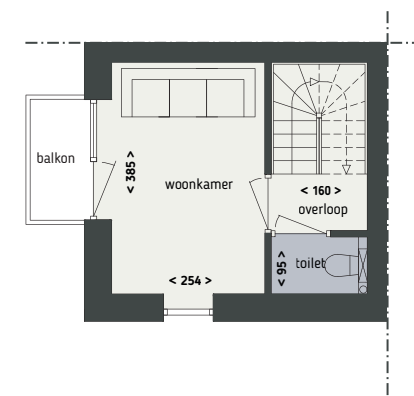
EERSTE VERDIEPING
