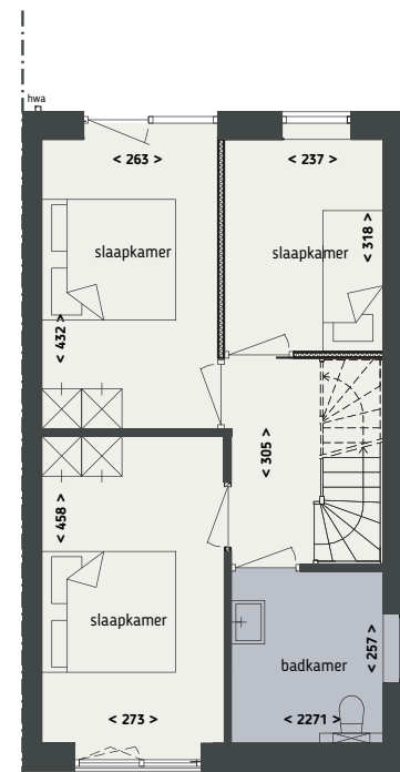
EERSTE VERDIEPING
