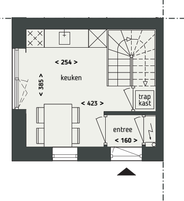
BEGANE GROND
